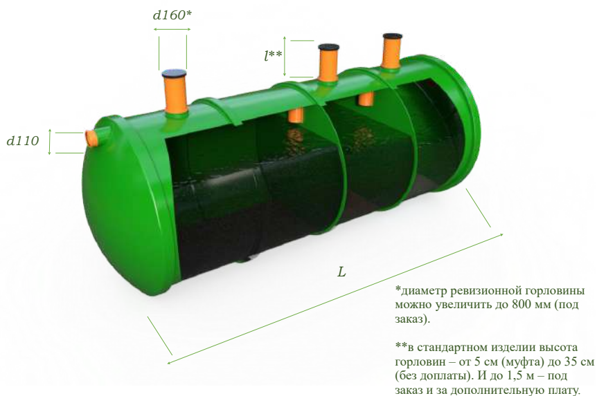
Рис 1. Устройство септика
