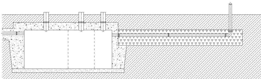
Рис. 6 Устройство впитывающей площадки
